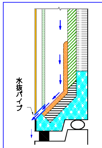
施工断面例
