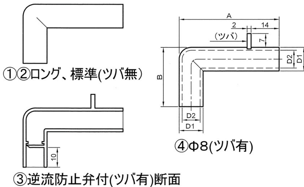
水抜きパイプL型寸法表
